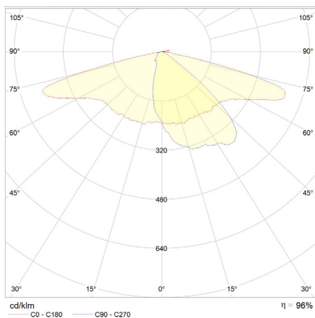
CREE XTE
