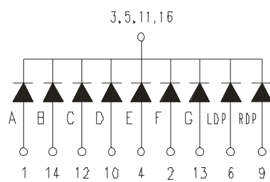
KPS-8102A
