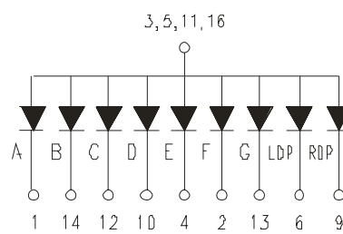
KPS-8102B
