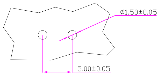
适配电路板尺寸
