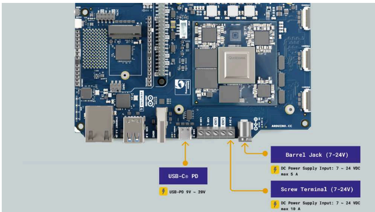
Input Power Options
