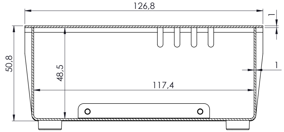
KESIT A-A
