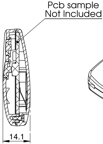
KESIT A-A
