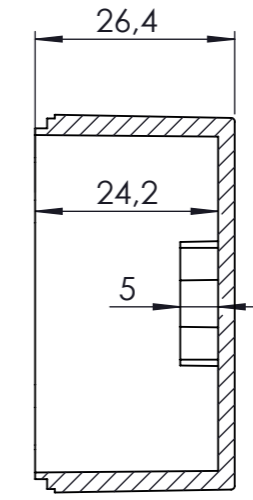
KESIT A-A
