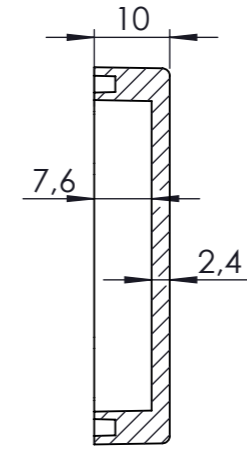
KESIT A-A
