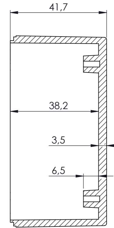
KESIT A-A
