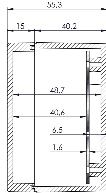
KESIT A-A
