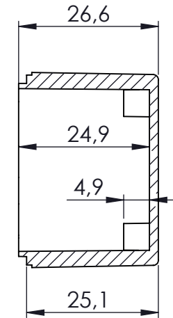
KESIT A-A
