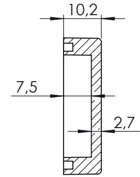
KESİT A-A
