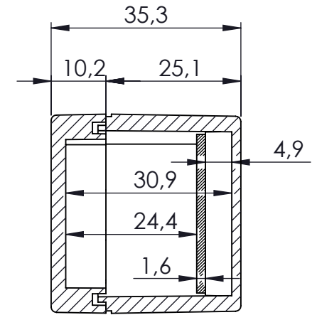
KESIT A-A
