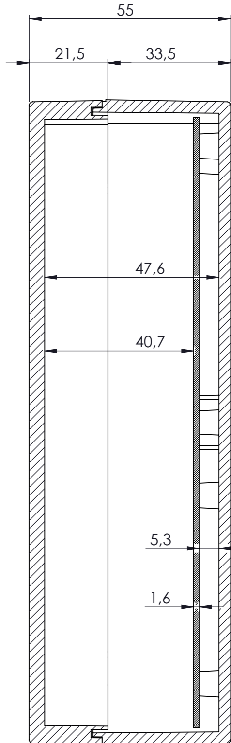
KESIT A-A
