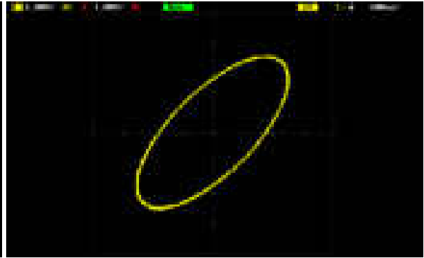
Faz açısı 45°
